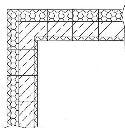
Grundriss: Eckausbildung
