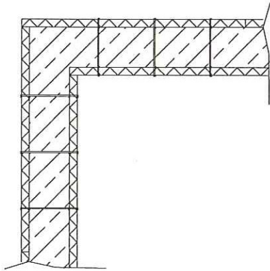
Grundriss: Eckausbildung
