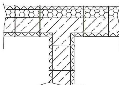
Grundriss: Einbindung Innenwand
